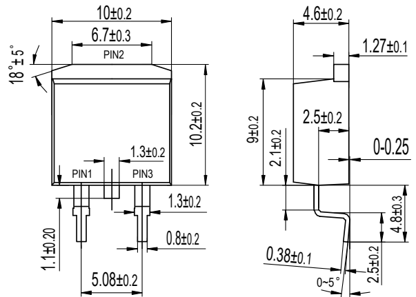
TO-263(D 2 PAK)
