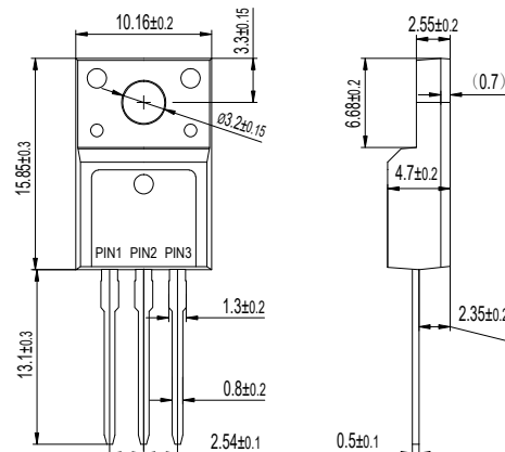
ITO-220AB
