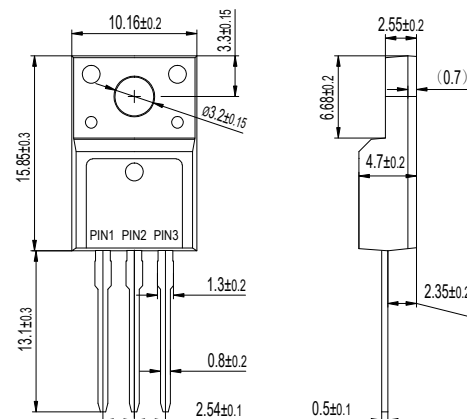
ITO-220AB
