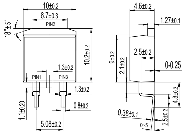
TO-263(D 2 PAK)
