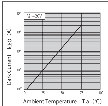
暗電流一周圍温度特性 (代表例)
